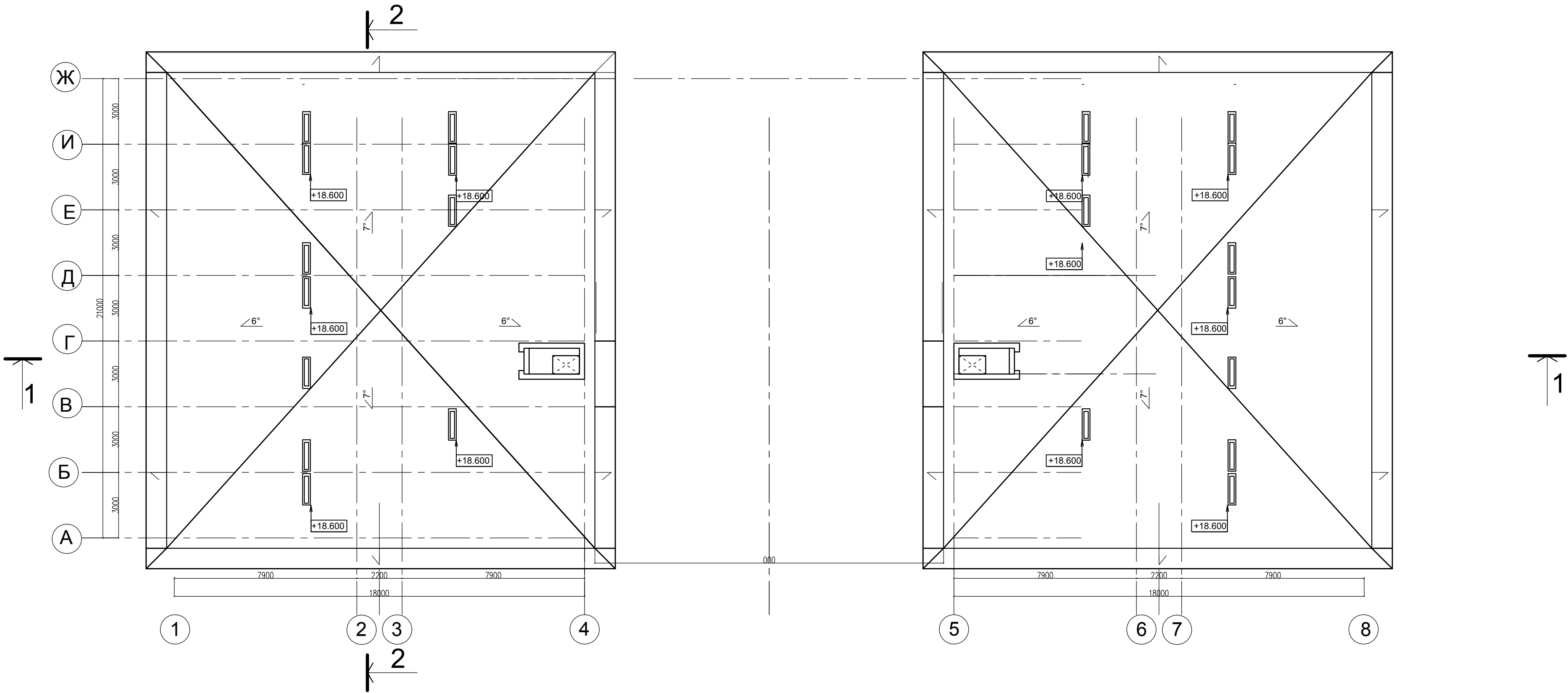
План кровли М1:200
